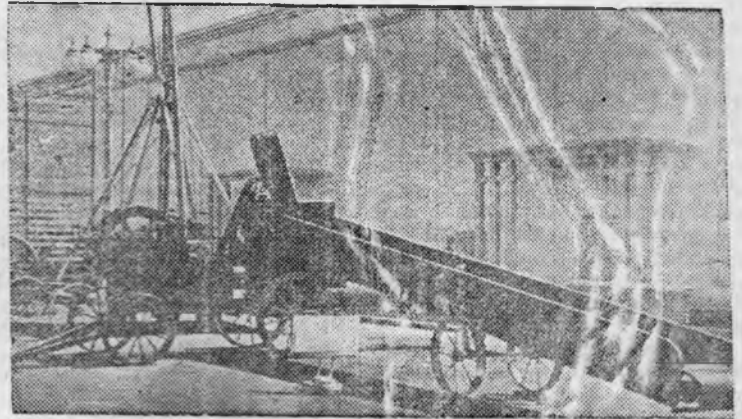
Новый сепной пресс «ВК-35х45» для прессовки сена в тюки (производство завода имени Коллющенко в г. Челябинске). Производительность 5 тонн в час.
