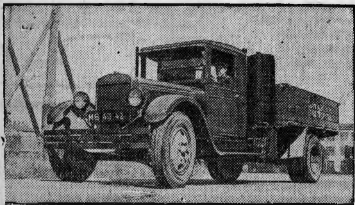
НА СНИМКЕ; Трехтонная машина ЗИС-5, с газогенератором Г-23.
