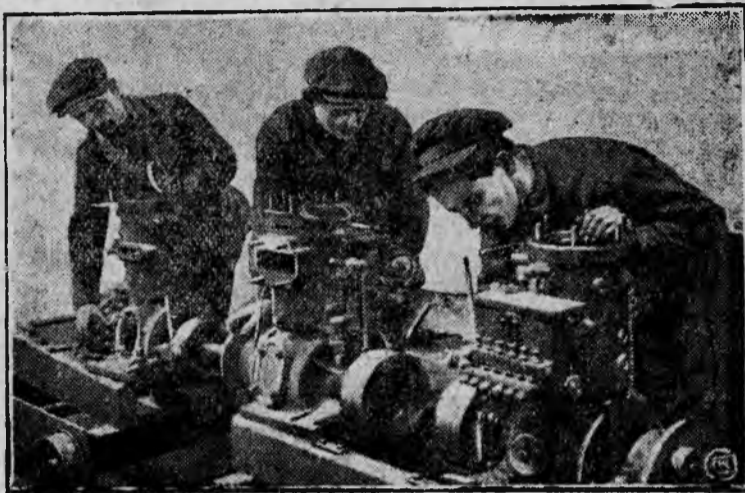
Завод „Победа Металлиста“—единственный в Союзе завод, изготовляющий нефтяные двигатели легкого типа для рыбацких судов. В связи с приближением весенней путины изготовление двигателей идет ударными темпами. Двигатели изобретены советским инженером т. Ремпелем и по сравнению со старыми двигателями дают экономию топлива и металла больше 50 проц. НА СНИМКА: Сборка двигателя.
